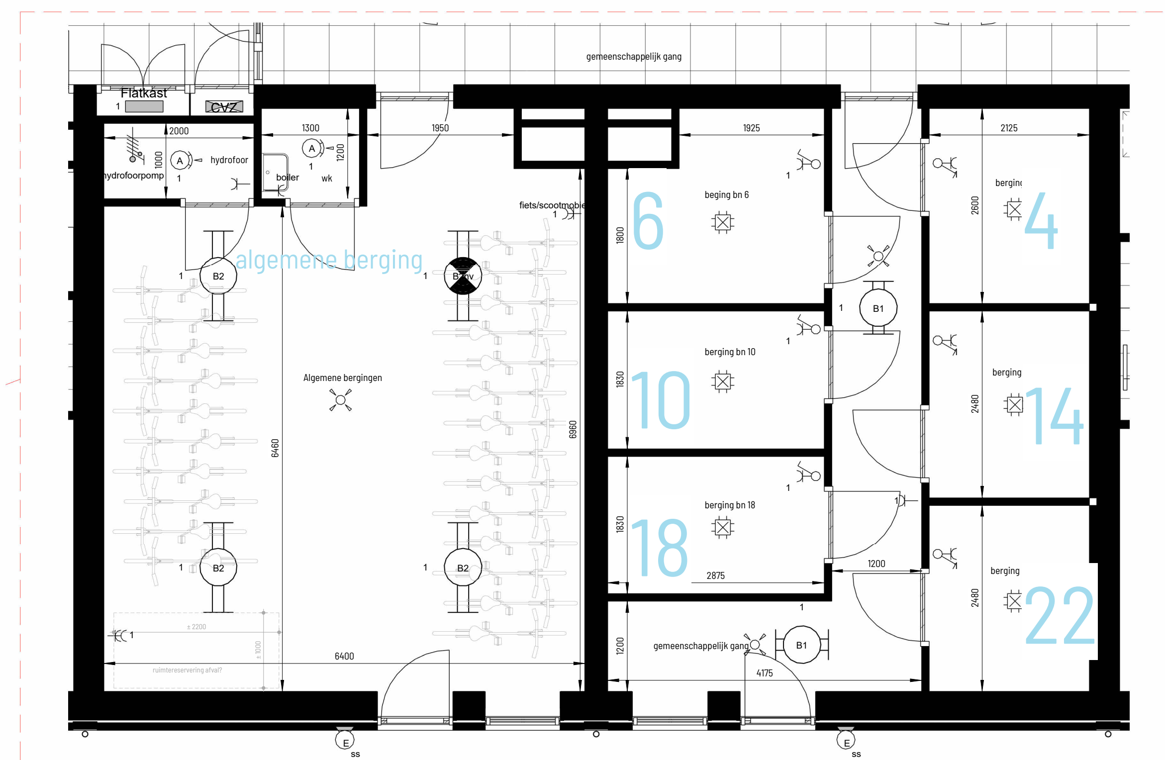
algemene ruimte + bergingen 1:50
